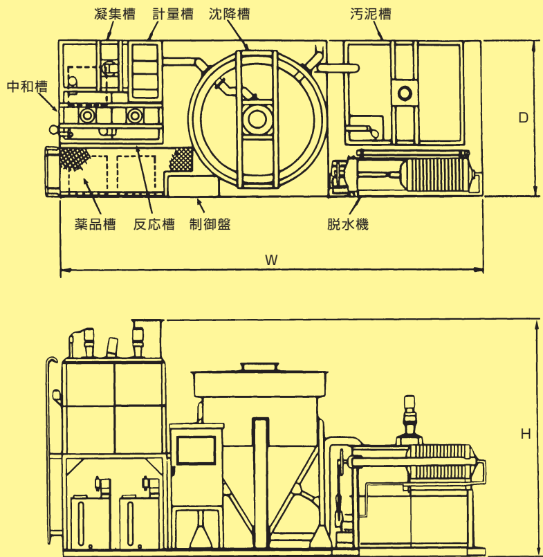
外観図
